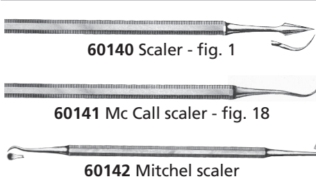
60142 Mitchel scaler
